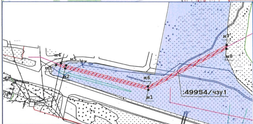
Расчет геоанных, вычисление площади СК МСК-50 зона-2
